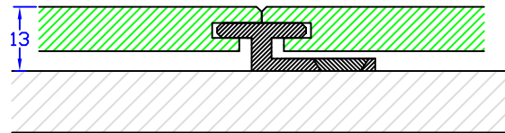
Plattenstoss Zwischenbefestigungsleiste
